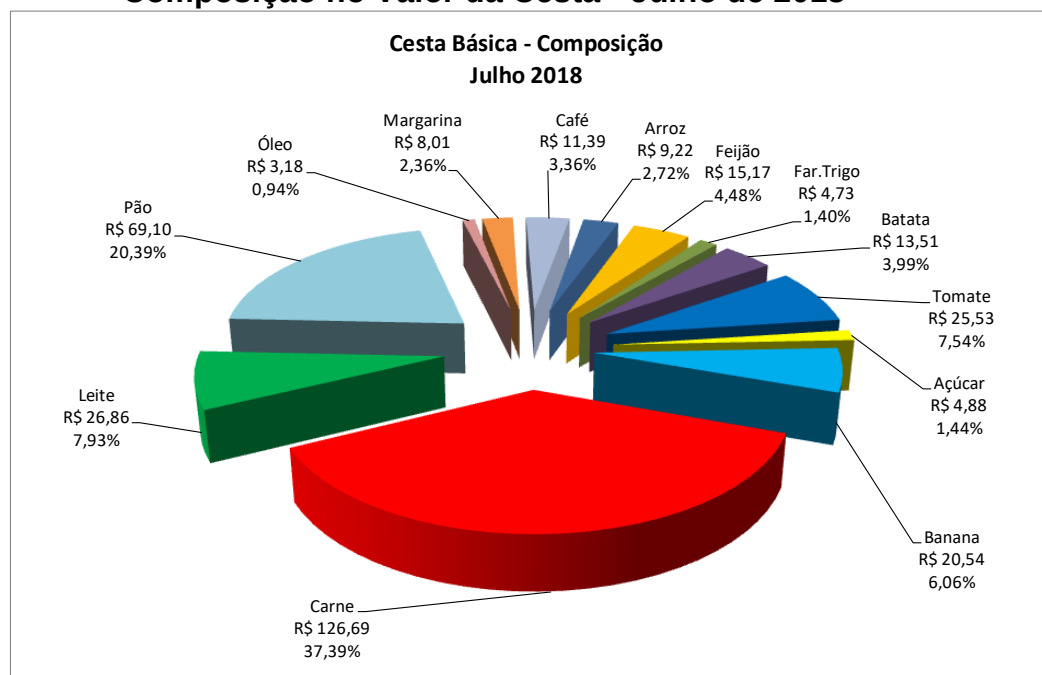
Gráfico 2. Cesta Básica de Alimentos de Uberlândia - Produtos Composição no Valor da Cesta - Julho de 2018
